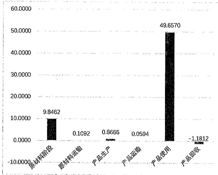
图 4.2-1 1 只 A 级单相费控智能电能表产品碳足迹各过程排放量 (kgCO 2 eq)
